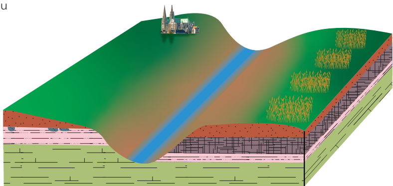
Coupe géologique de Chartres.
